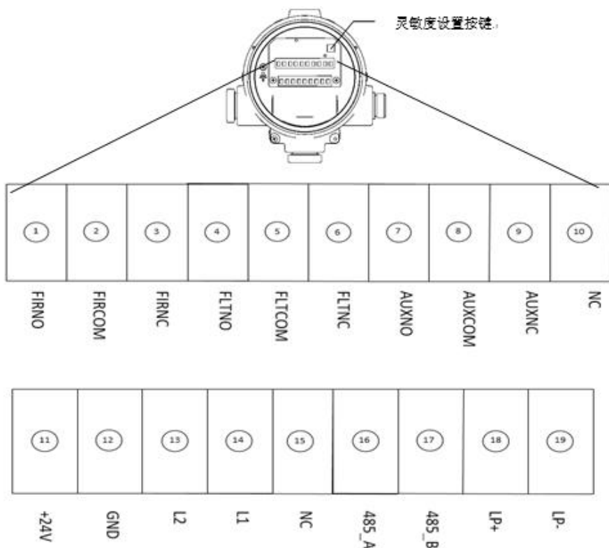
图 1 端子接线图
