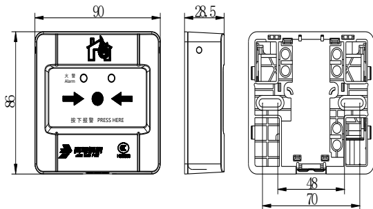
图 1 外形及尺寸图
