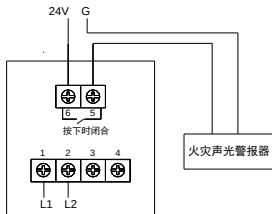
图2 端子接线图
