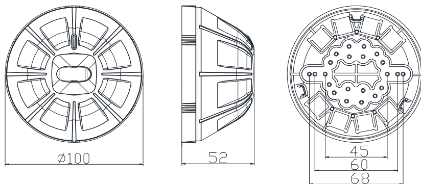
图 1 外形及安装尺寸图（不带支架）
