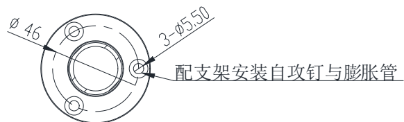
图 1 外形及安装尺寸图（不带支架）
