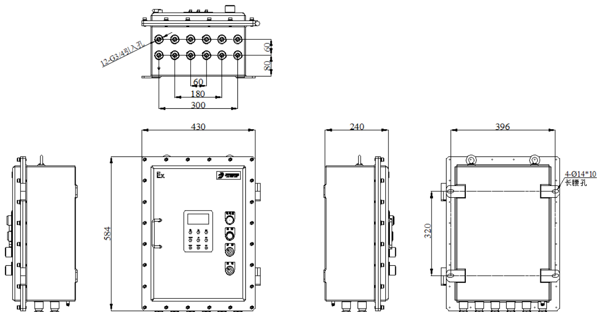
图 2.1 外形尺寸图
