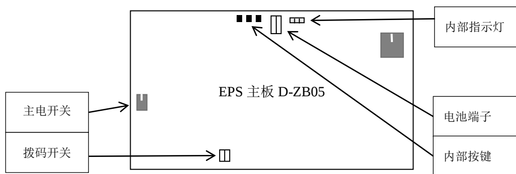
图 5.1 拨码开关及主备电开关位置示意图
