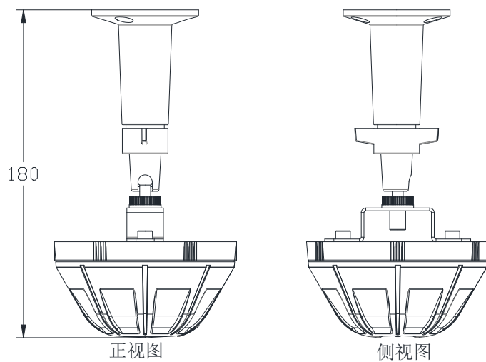
图 2 外形及安装尺寸图（带支架）
