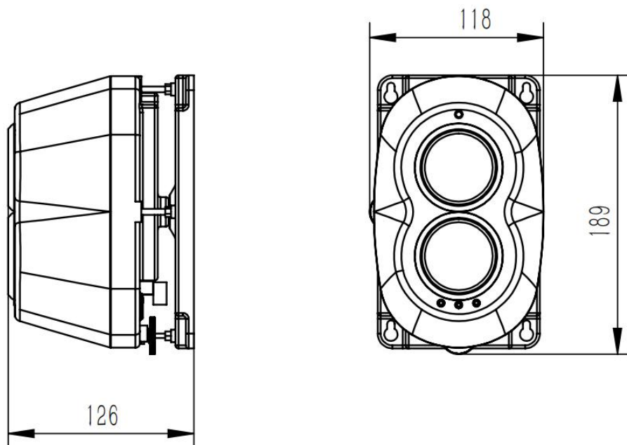
图 1 外形及安装尺寸图 (单位: mm)
