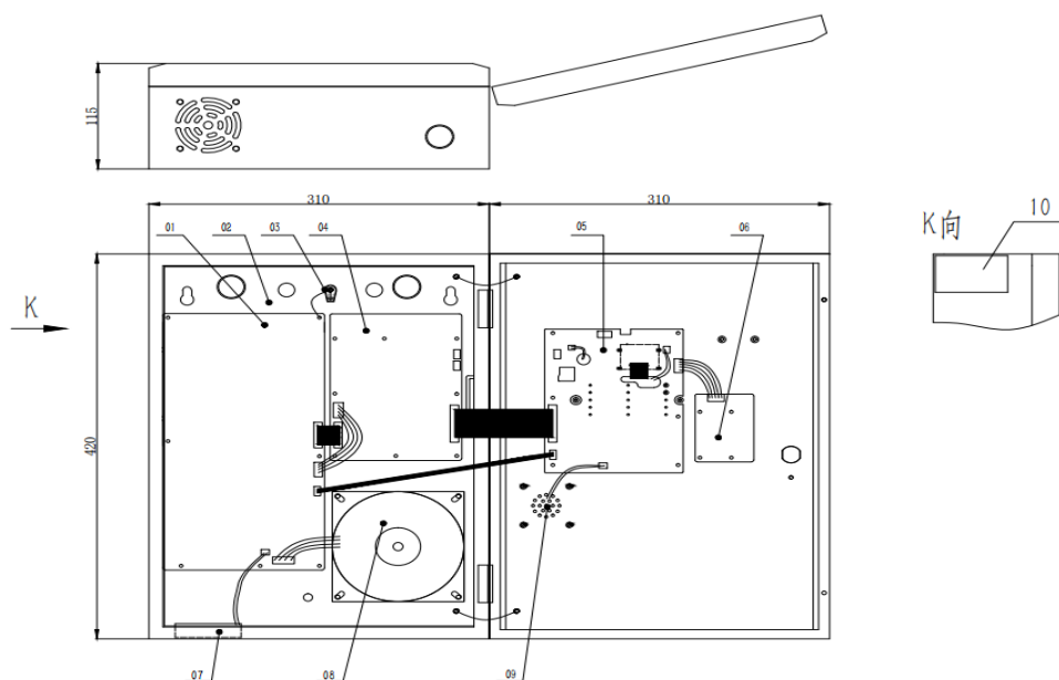
图 3-1 箱体（单位：mm）
