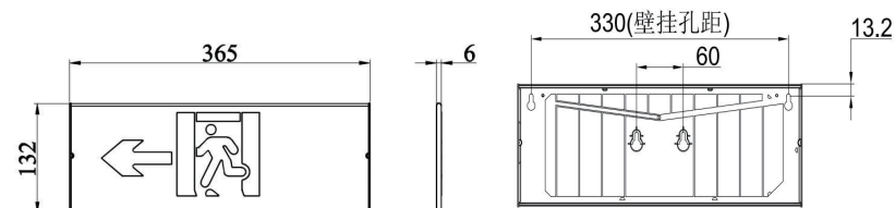
c) 不锈钢背板款吊装灯具
