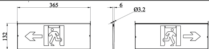
b) 单面壁挂灯具
