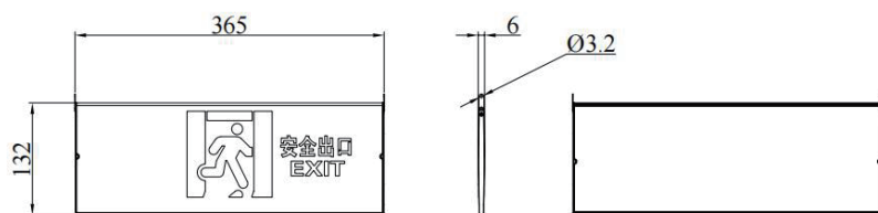
c) 不锈钢背板款吊装灯具
