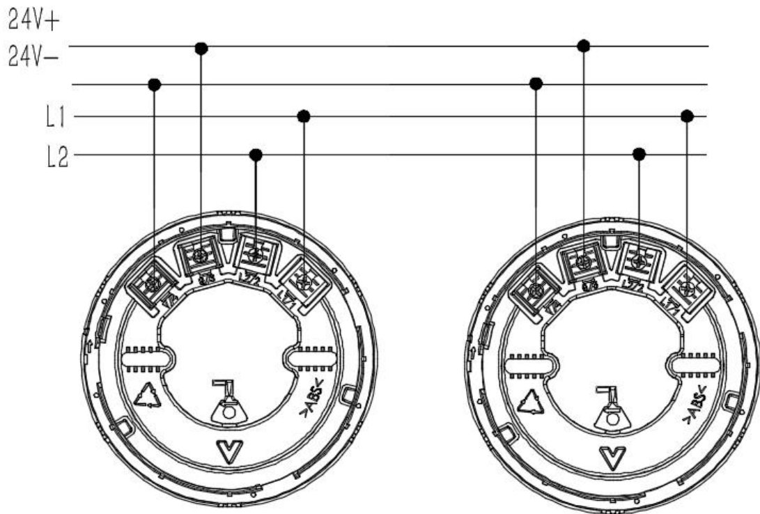
图 2 接线图例
