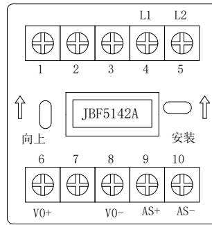
图 2 端子图
