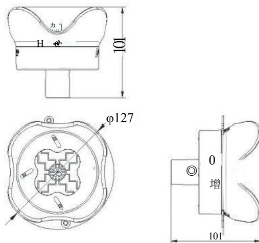
图 1 外形尺寸图
