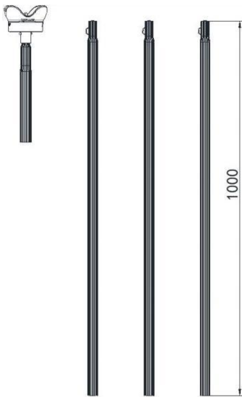
图 2 外形尺寸图
