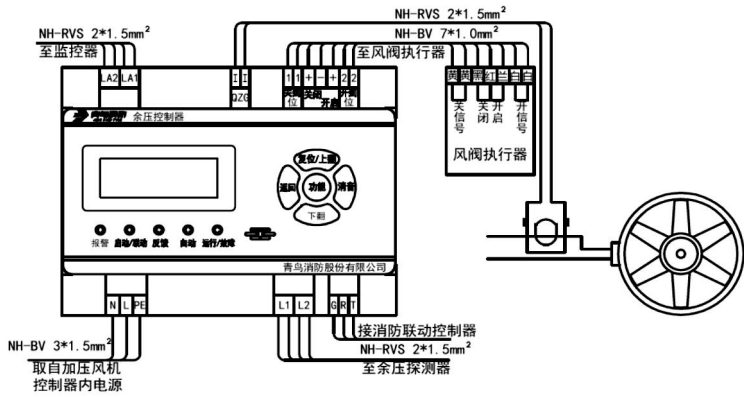
图 7 控制器接线图
