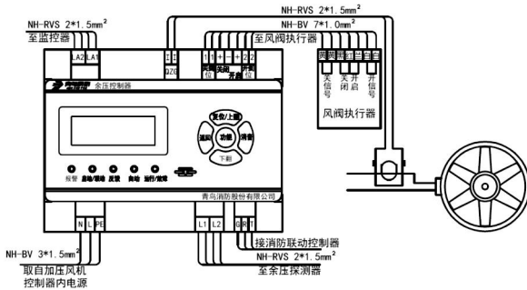
图 33 接线示意图
