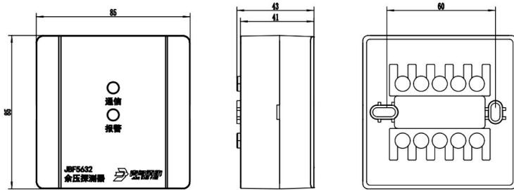
图 8 JBF5632 探测器尺寸及安装孔位示意图
