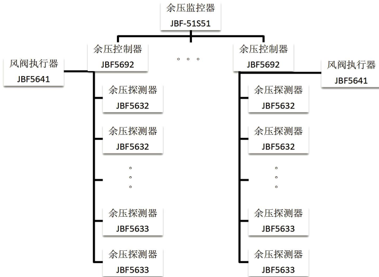
消防应急疏散余压监控系统框图
