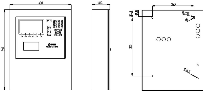
图 26 监控器外形及安装尺寸
