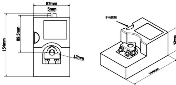
图 34 外形尺寸及安装尺寸图
