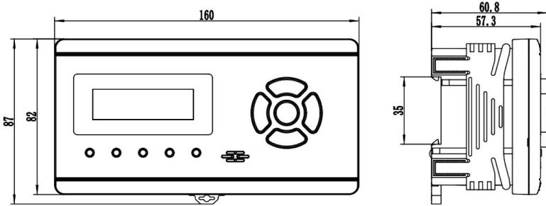
图1 控制器外形尺寸
