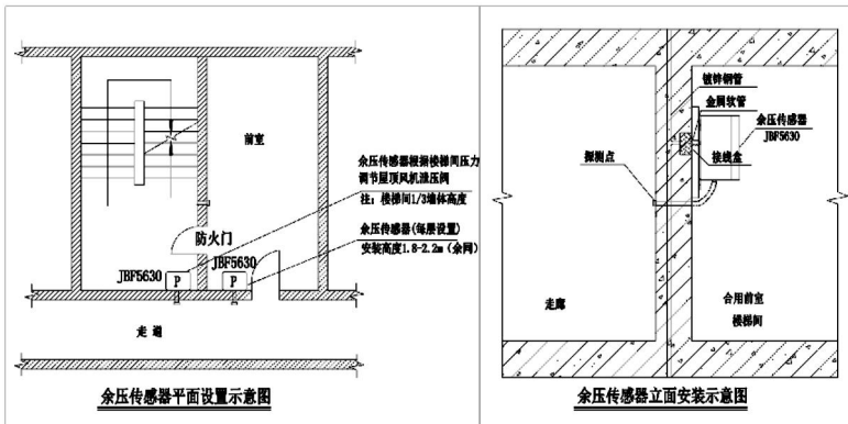
图 10 探测器安装示意图
