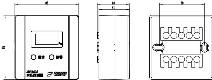
图 9 JBF5633 探测器尺寸及安装孔位示意图
