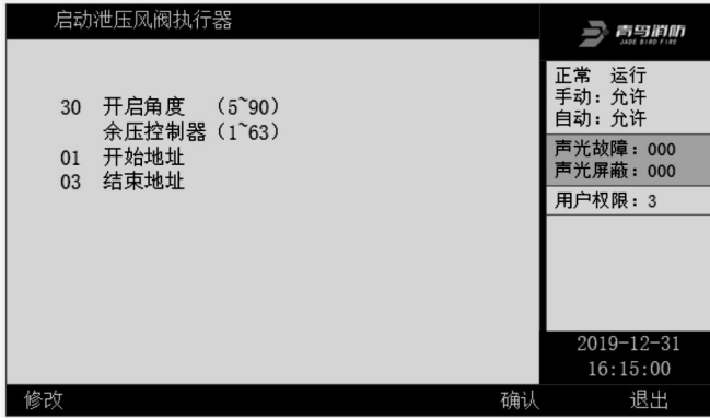
图 32 启动泄压风阀执行器界面
