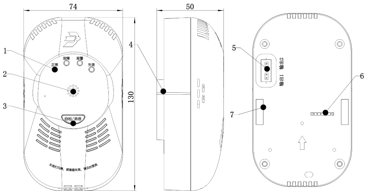
1. 指示灯区域 2. 出音口区域 3. 按键区域 4. 对齐刻度 5. 输出区域 6. 联网区域 7. 挂板滑槽
