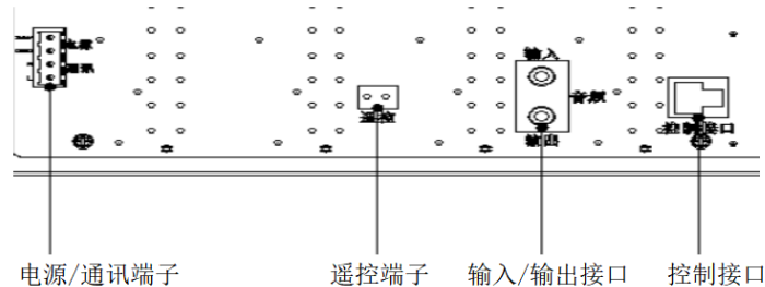
图4-1接线示意图
