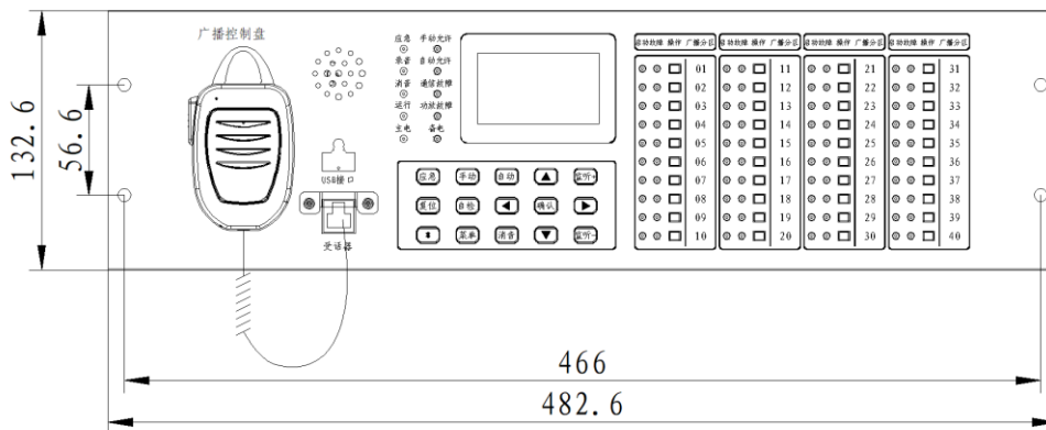
图 3-1 箱体（单位：mm）
