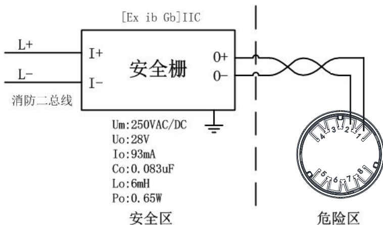
图 4 接线图例
