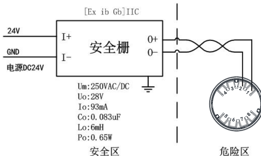
图 5 接线图例
