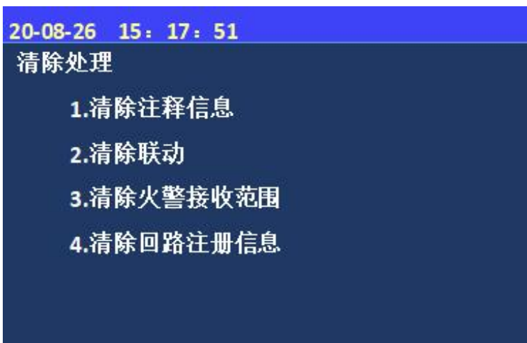
图4.4.2 清除处理
