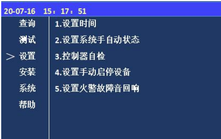
图4.2设置菜单
