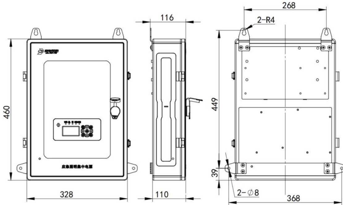
J-D-AC(DC36V/0.25kVA)-01L 外形尺寸示意图
