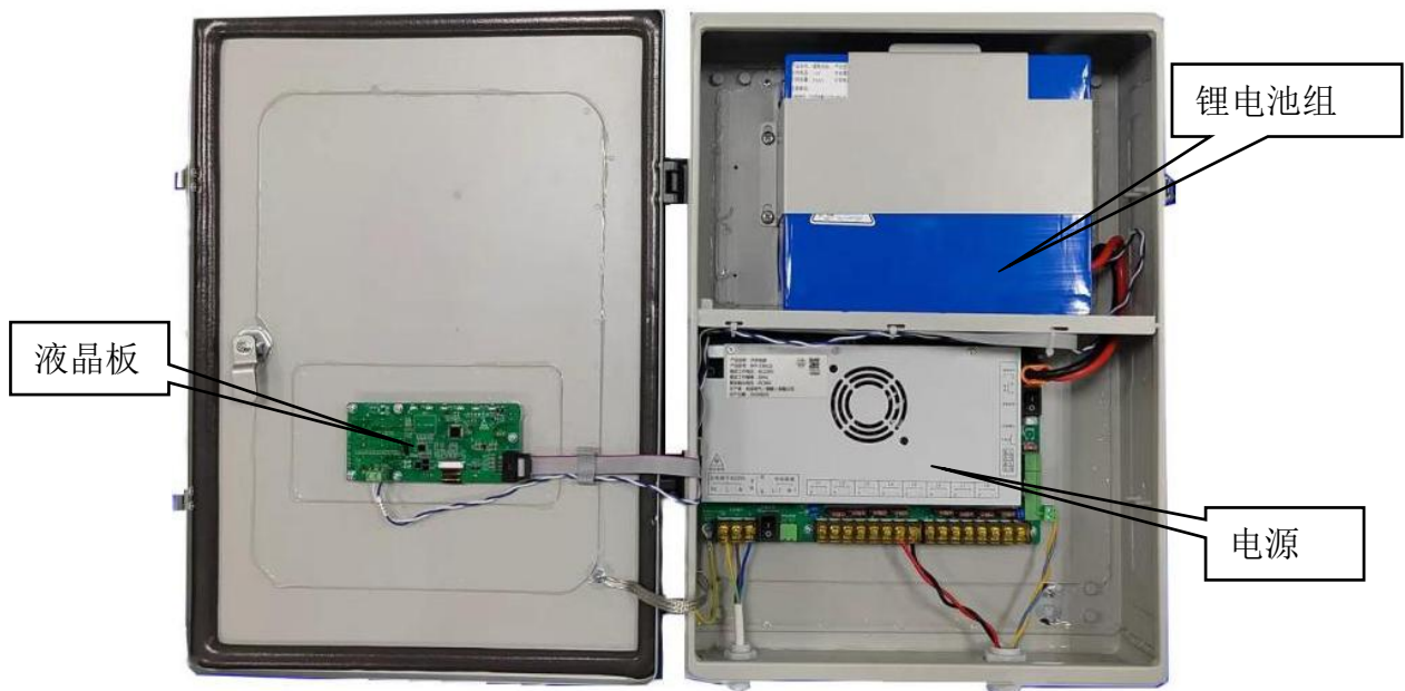
J-D-AC(DC36V/0.25kVA)-01L 内部结构图
