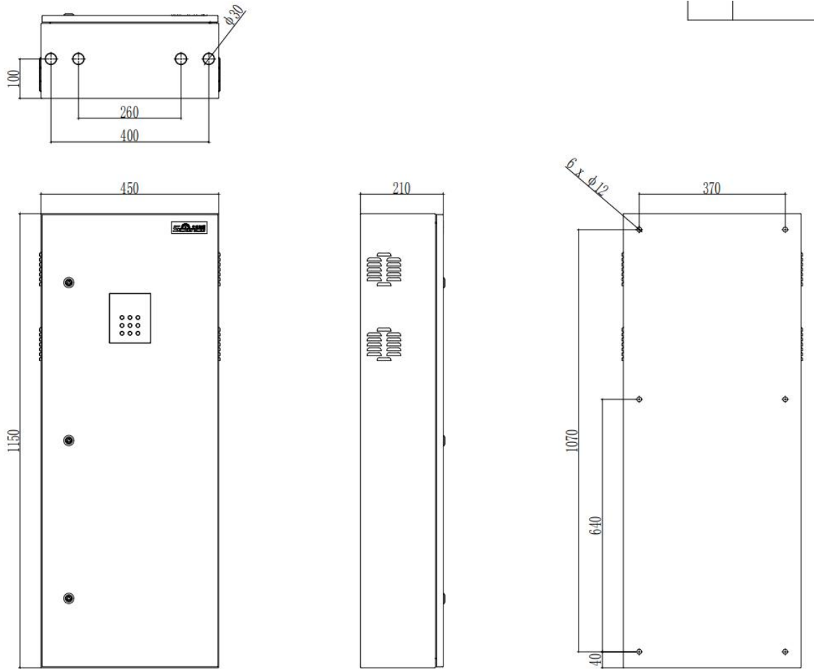
图 2.1 外形尺寸图
