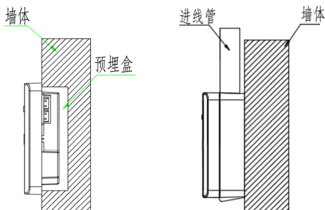
图 3、暗装方式图 4、明装方式
