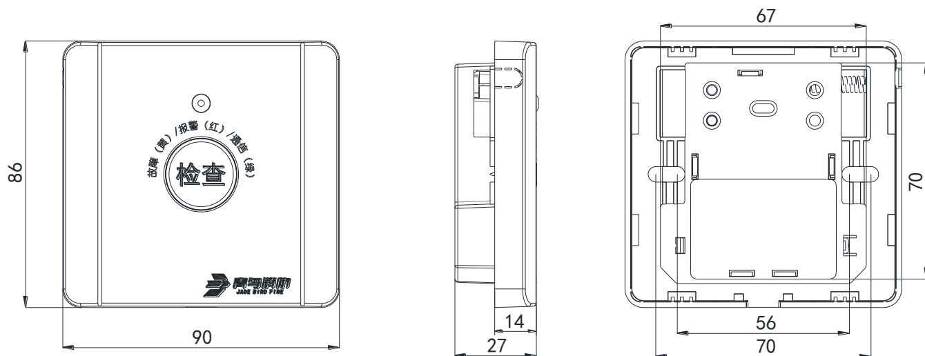
图 2 外形及尺寸图 (不含底座)
