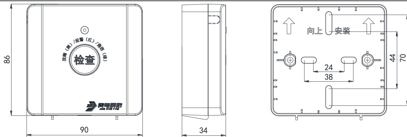
图 1 外形及尺寸图 (含底座)
