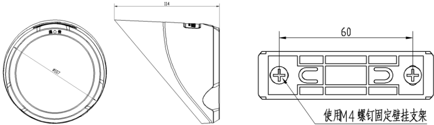
灯具尺寸
