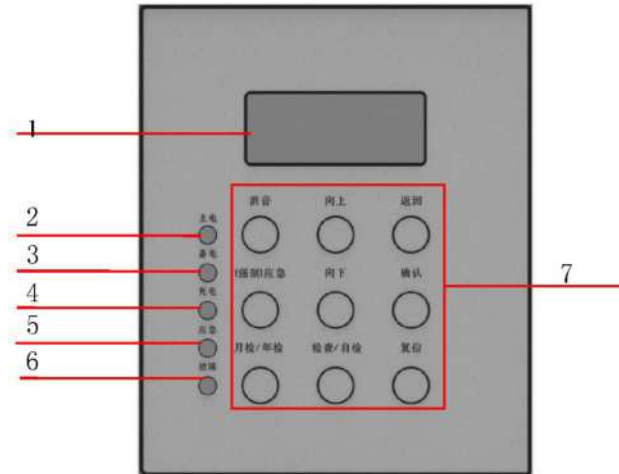
图 4.1 操作面板
