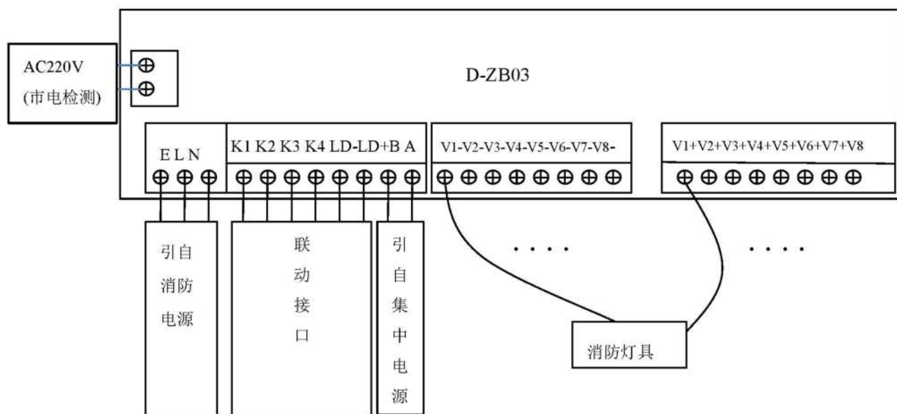
图 3.1 应急照明控制器接线示意图
