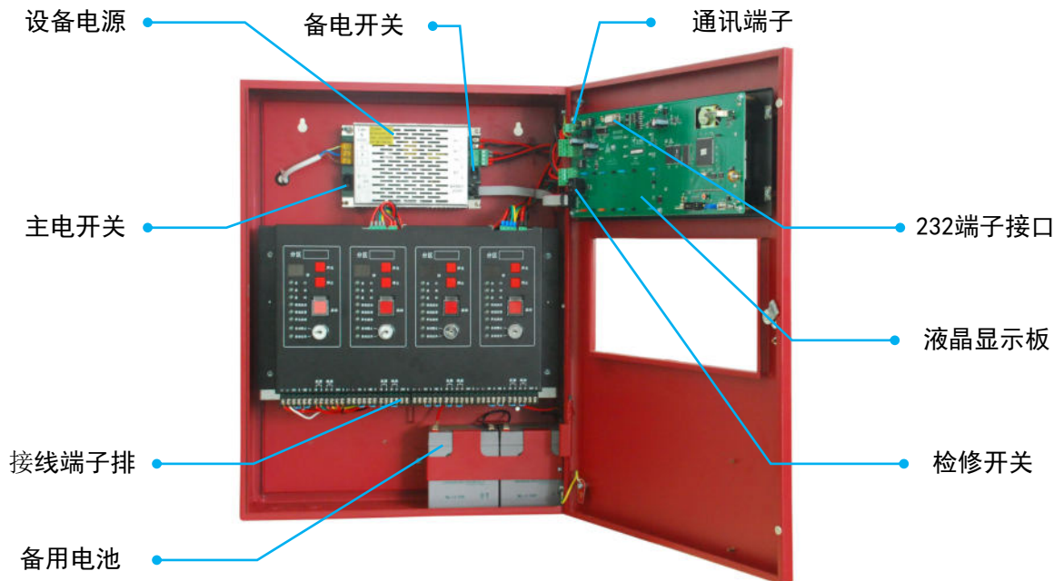
内部部位图
