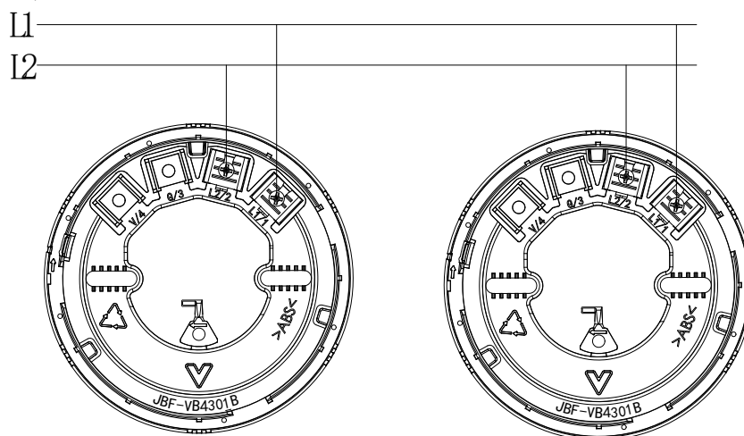
图 2 接线图例
