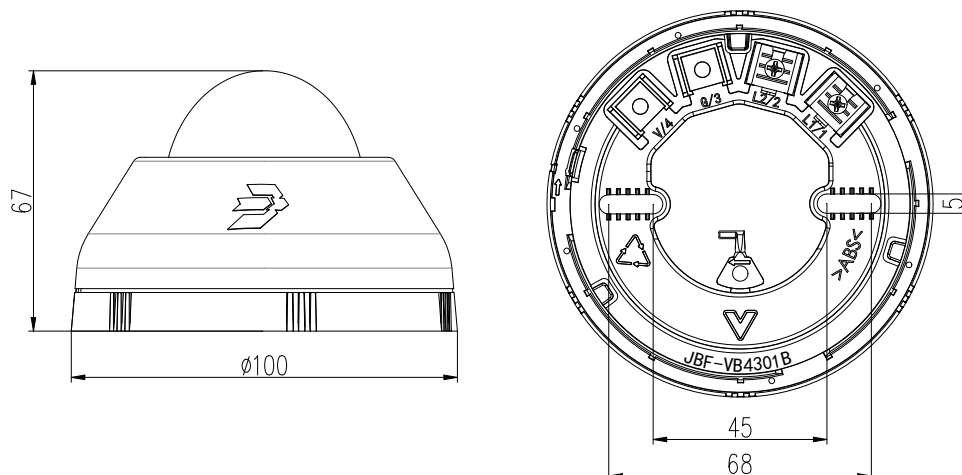
图 1 外形及尺寸图
