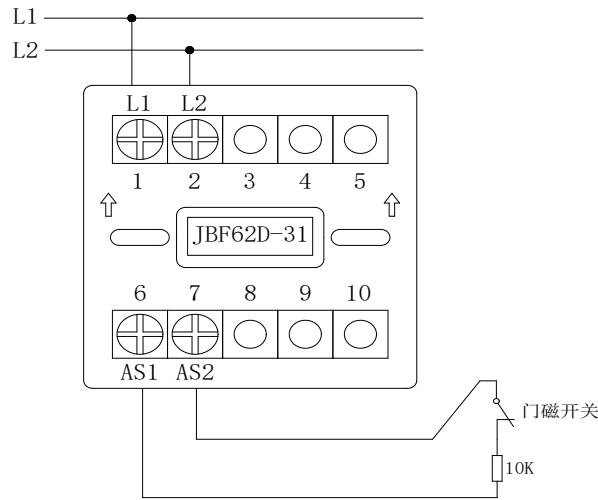
图 3 接线示意图
