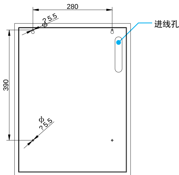
安装尺寸图
