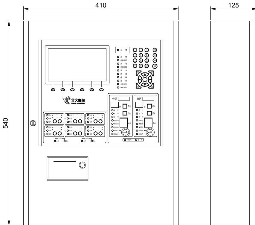
外形尺寸图
