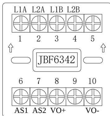
图 2 端子图
