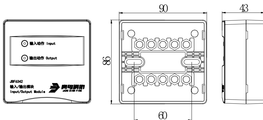
图 1 外形及安装尺寸图
