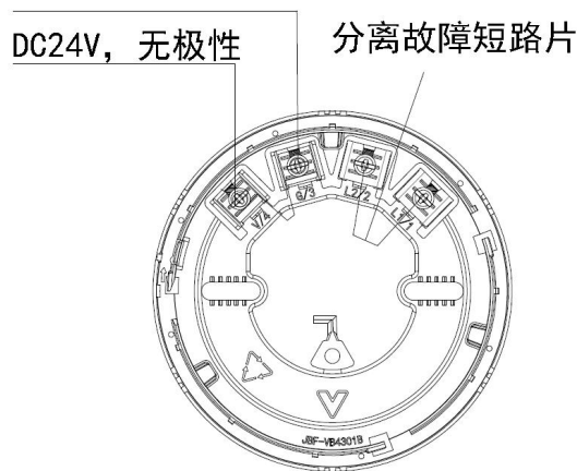
图 2 端子图
