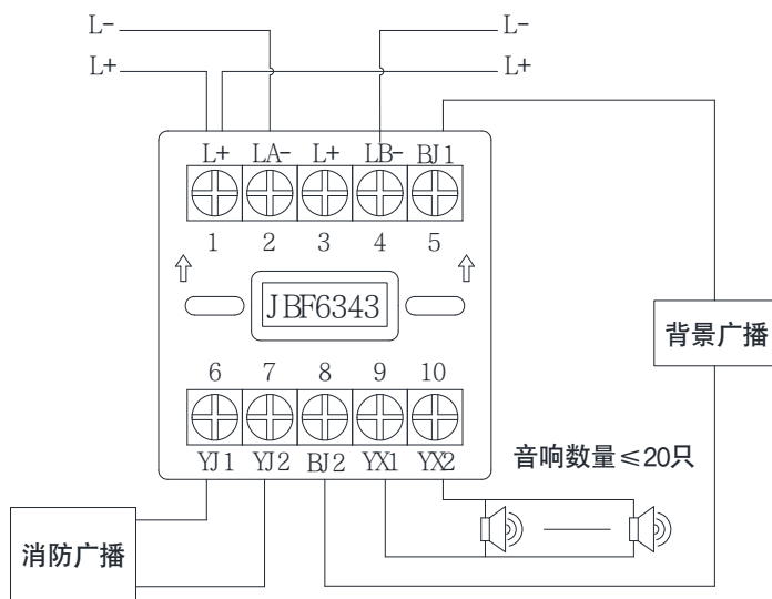
图3 接线图
