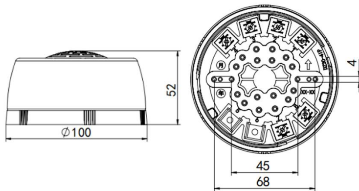
图 1 外形及安装尺寸图
