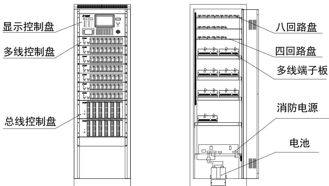
立柜型控制器结构介绍
