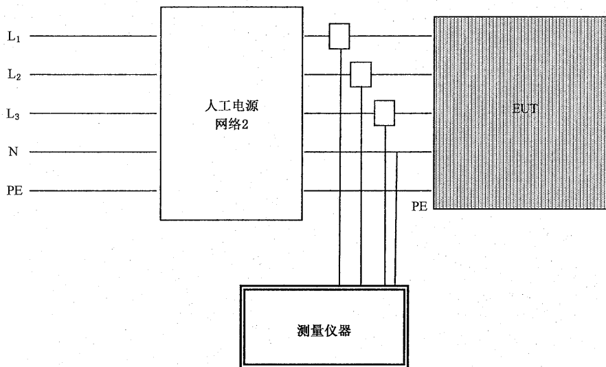
b) 三相测量布置
