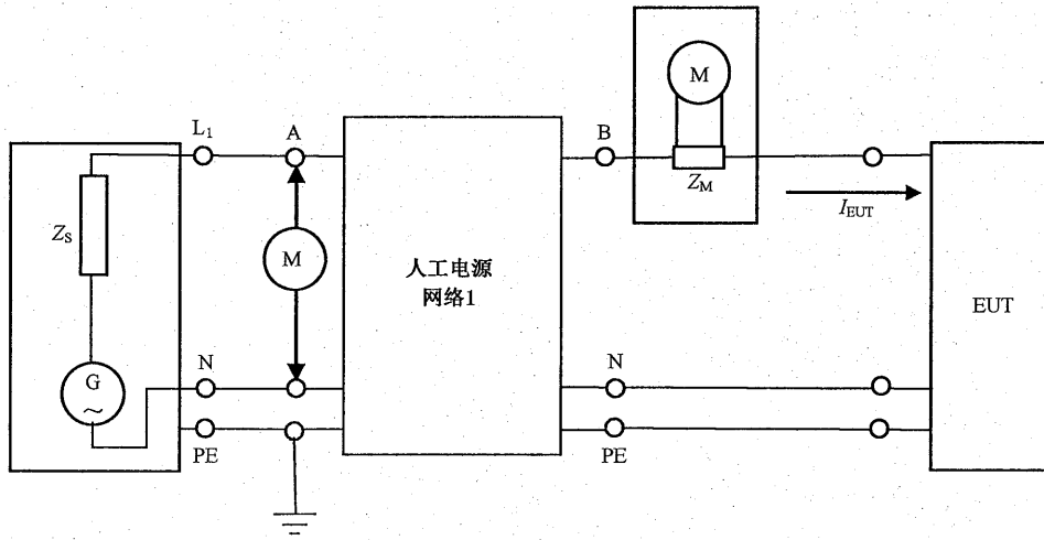
a) 单相测量布置
