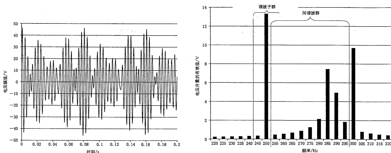
图 C.5 287 Hz 的间谐波以及 5 次和 6 次谐波
