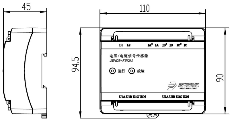
4JBF62P-ATV2A1 结构尺寸图
