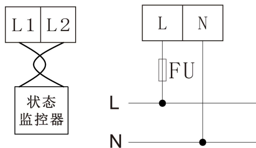
JBF62P-ASV1 接线图
