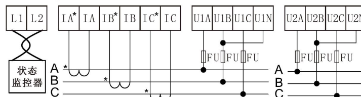
JBF62P-ATV2A1 三相三线接线图
