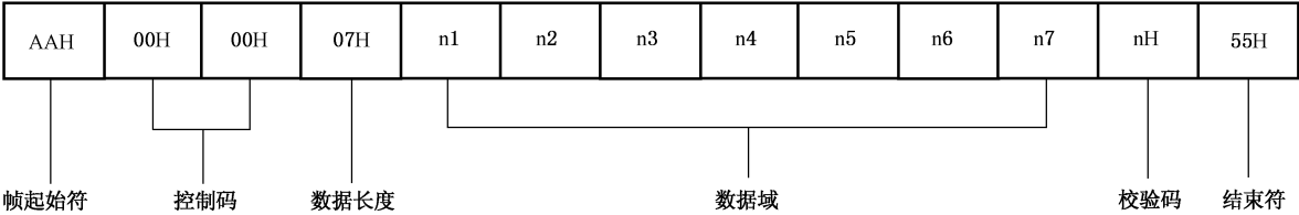
图 A.5 应答帧(1)格式
