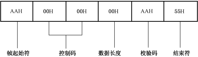
图 A.4 请求帧(1)格式
