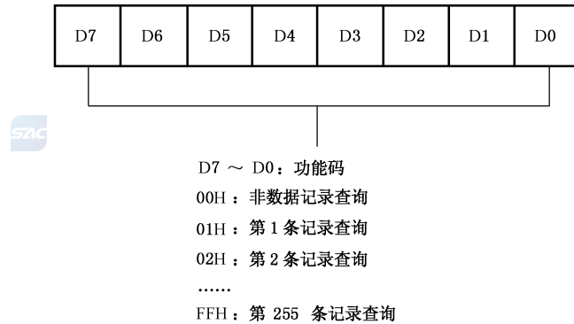
图 A.2 控制码 C1 格式
