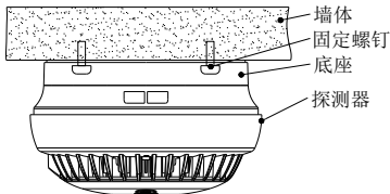
图 3 报警器螺丝安装示意图
