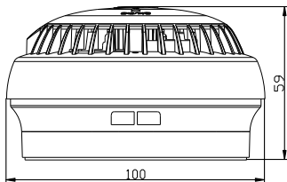
图1 外形尺寸示意图
