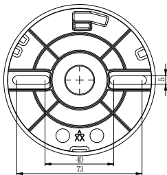
图2 底座示意图
