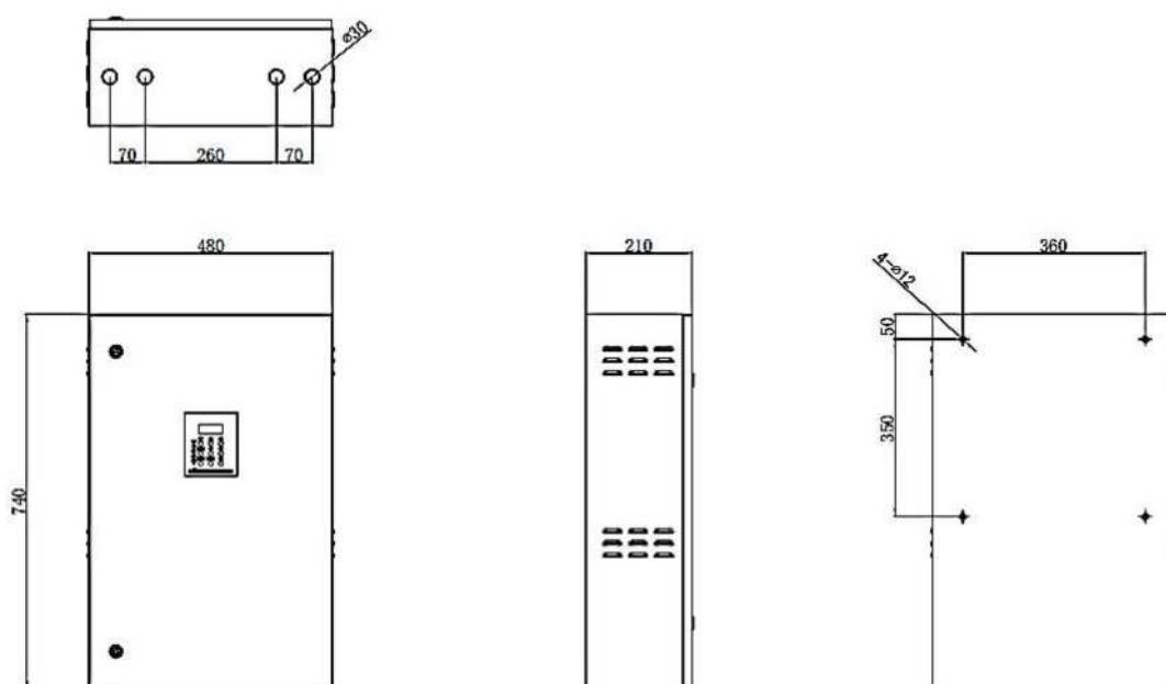
图 2.1 外形尺寸图
