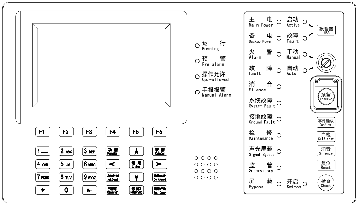
显示盘面板图
