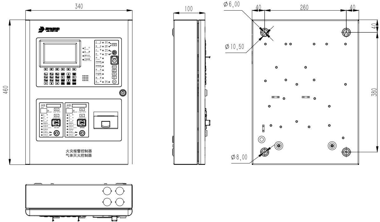
控制器尺寸图
