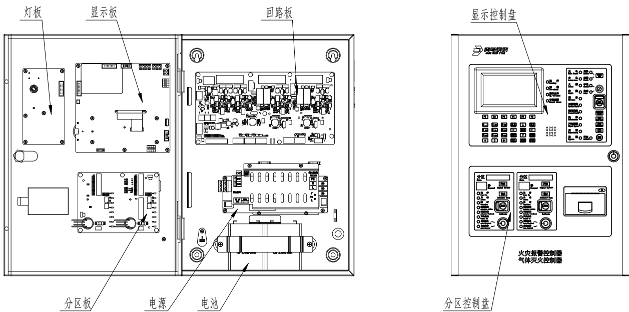
控制器结构介绍
