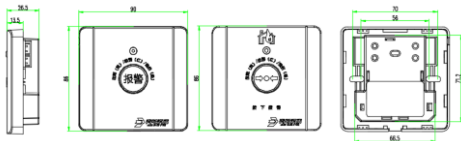
图 2 外形及尺寸图（不含底座）
