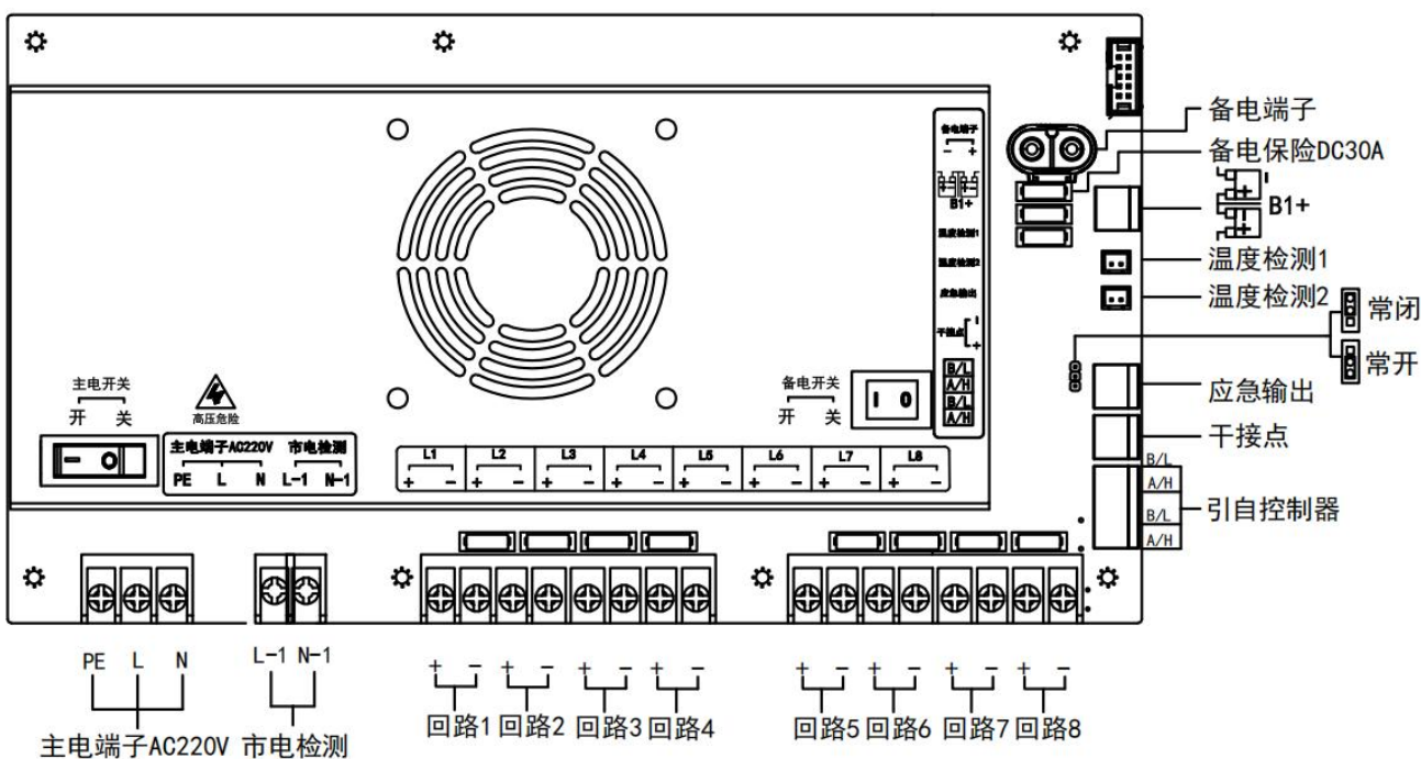
JF-D-AC(DC36V/1.0kVA)-DA120(65) 接线端子示意图
