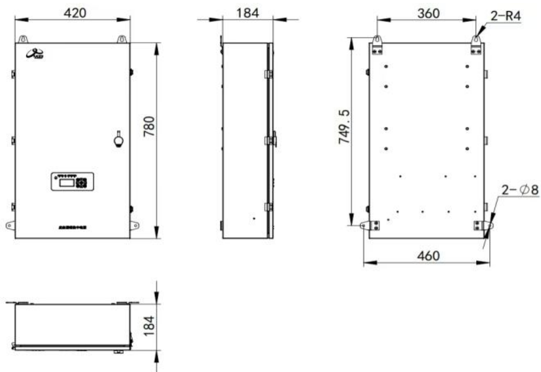
JF-D-AC(DC36V/0.6kVA)-DA112(65)外形尺寸示意图
