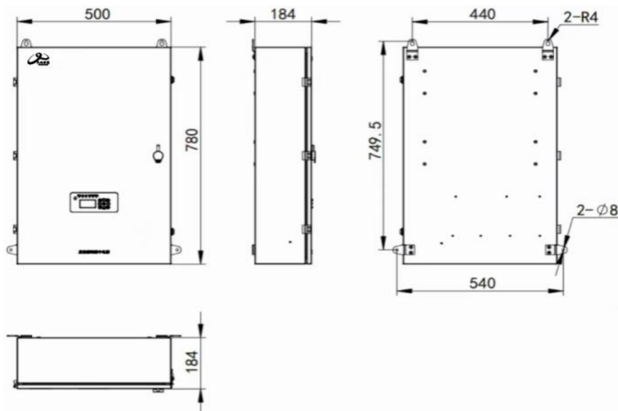
JF-D-AC(DC36V/1.0kVA)-DA120(65)外形尺寸示意图
