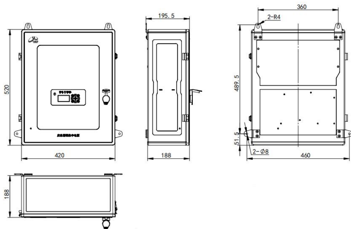
JF-D-AC(DC36V/0.45kVA)-DA109(65)外形尺寸示意图
