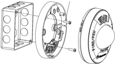
图 2. 安装底座
