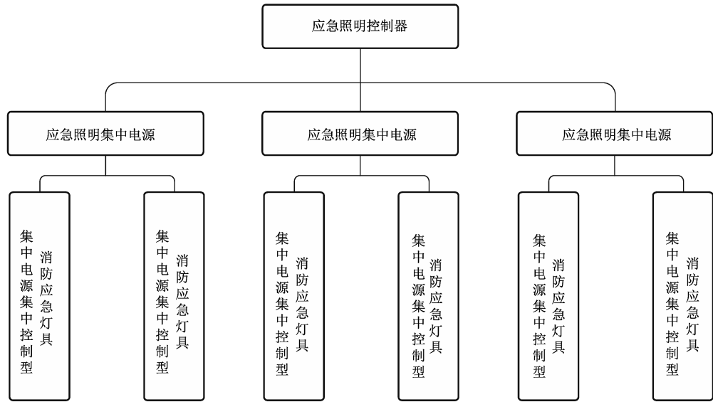
图 A.1 集中电源集中控制型系统组成
