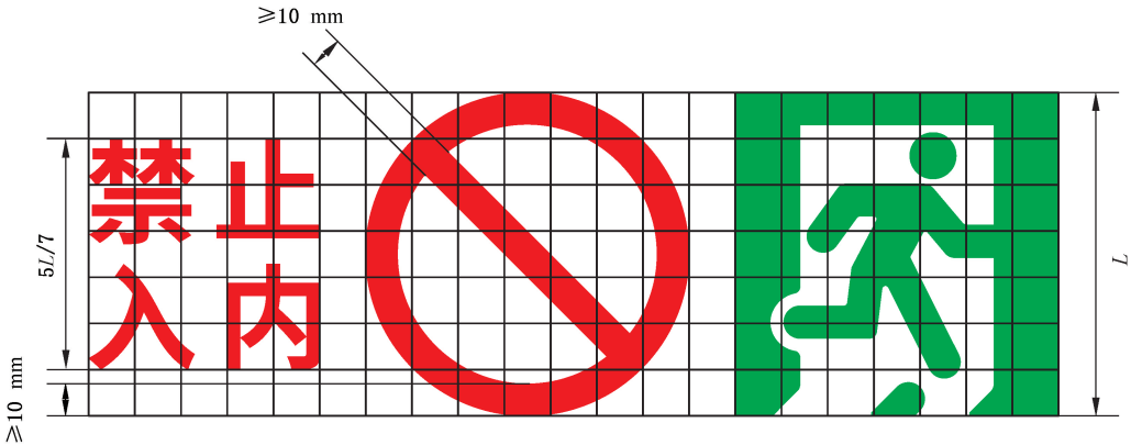
图 D.20 指示状态可变疏散出口标志图形
