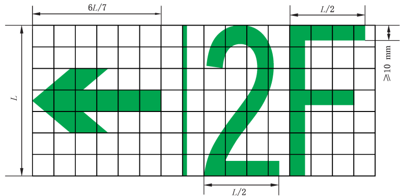
图 D.11 多信息复合标志图形
