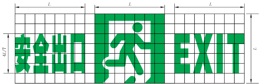
图 D.14 安全出口标志图形
