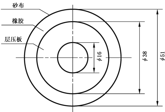
图 F.1 研磨轮
