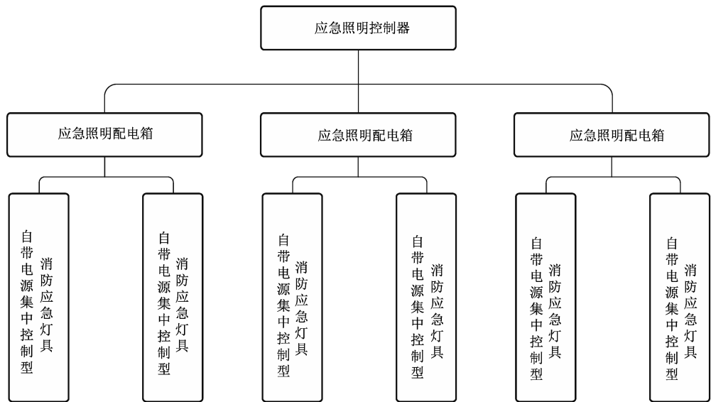
图 A.2 自带电源集中控制型系统组成
