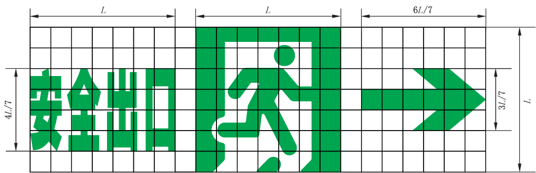
图 D.17 指示安全出口方向标志图形
