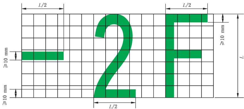
图 D.10 指示楼层指示标志图形
