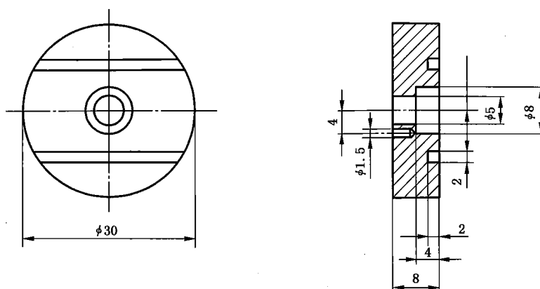
图 B.2 镉电极盘
