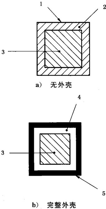
图 D.1 符合 6.3.5 和 6.6 浇封组件举例
