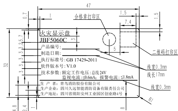
2:1 图样
