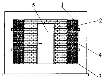
图 4 电缆隧道(双侧桥架)封堵断面图
