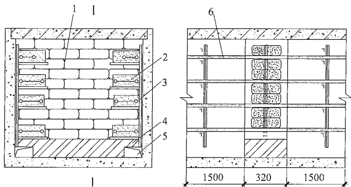
图 6 电缆沟防火墙
