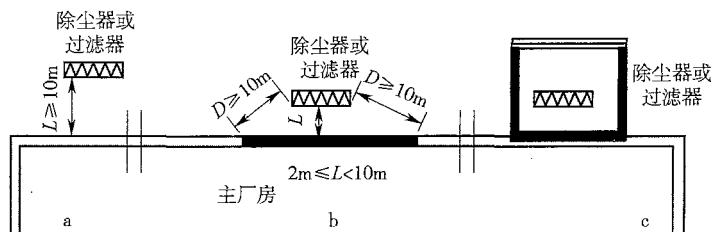
图 3 除尘器或过滤器的布置示意图
