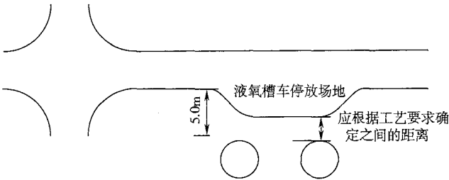
图 1 液氧槽车停放场地与储罐间距示意图
