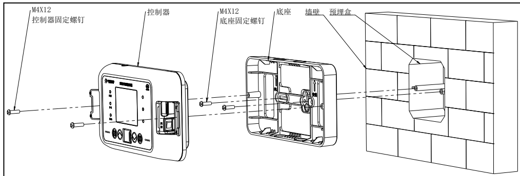
安装示意图
