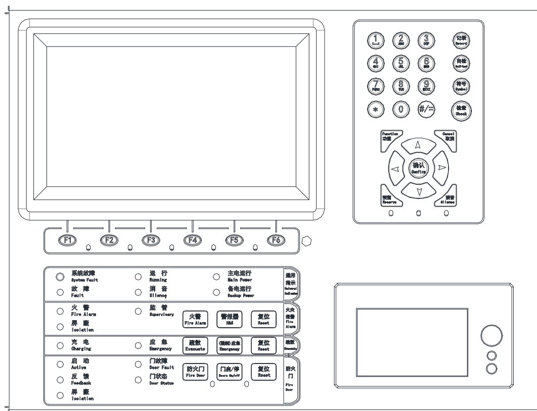
5-1 显示盘面板
