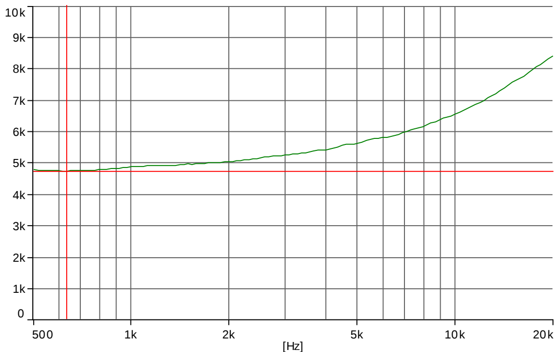
阻抗曲线
