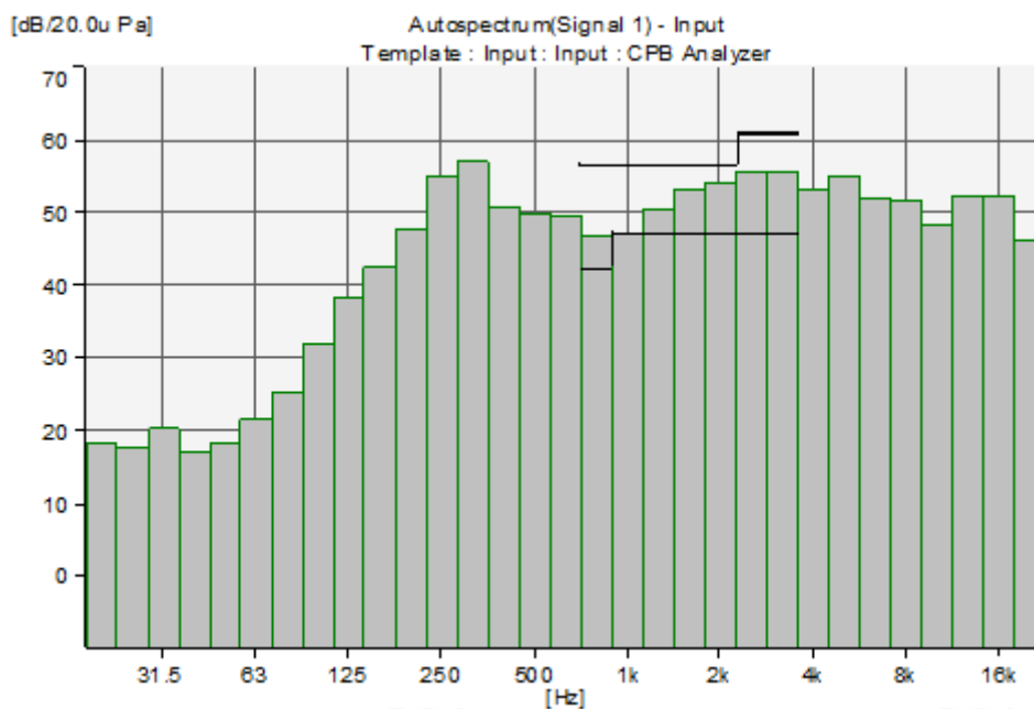
频率特性
