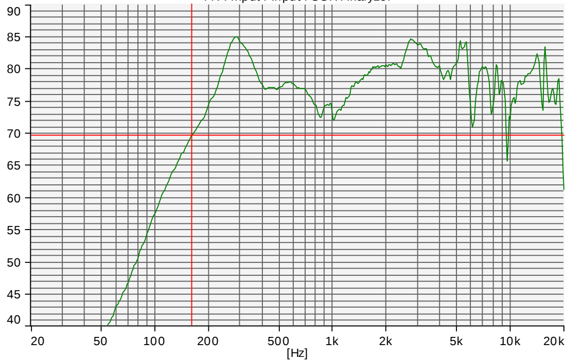
频响曲线
