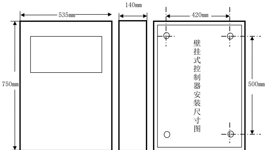
图 2- 1 JB-TB-JBF-11SF-S8 型控制器安装尺寸图
