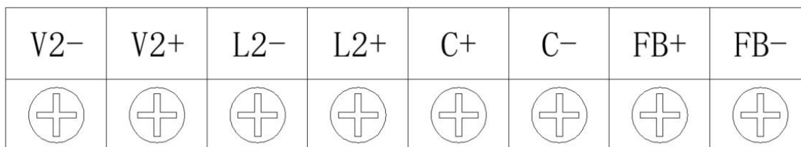
端子排示意图
