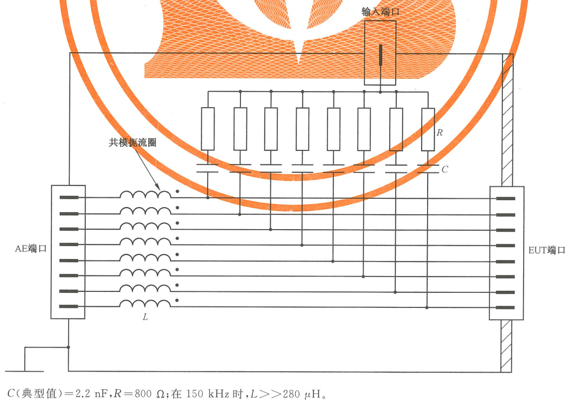
图 D.6 用于非屏蔽不平衡线的 CDN-AF8 简化电路图示例(见 6.2.2.4)
