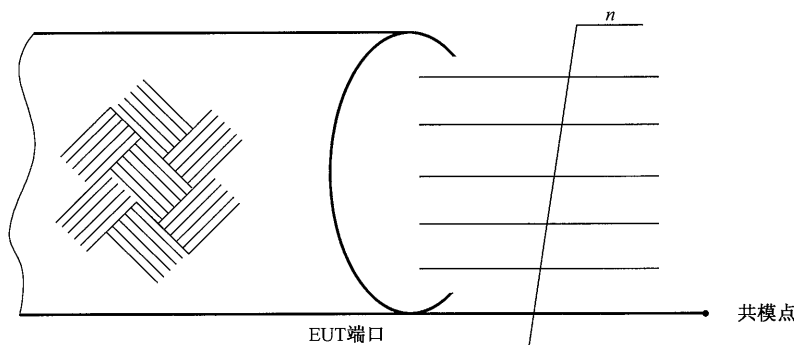
b) 屏蔽电缆的共模点定义
