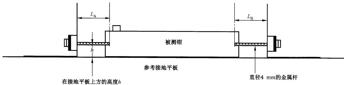
图 A.5 插入被测钳的试验夹具
