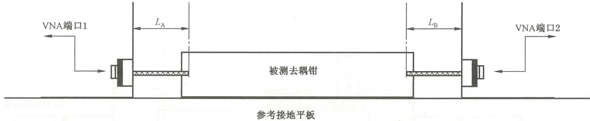
图 A.12 去耦钳特性的测量布置
